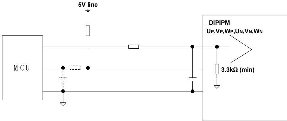
图 11 推荐的 MCU 输入输出接口电路
